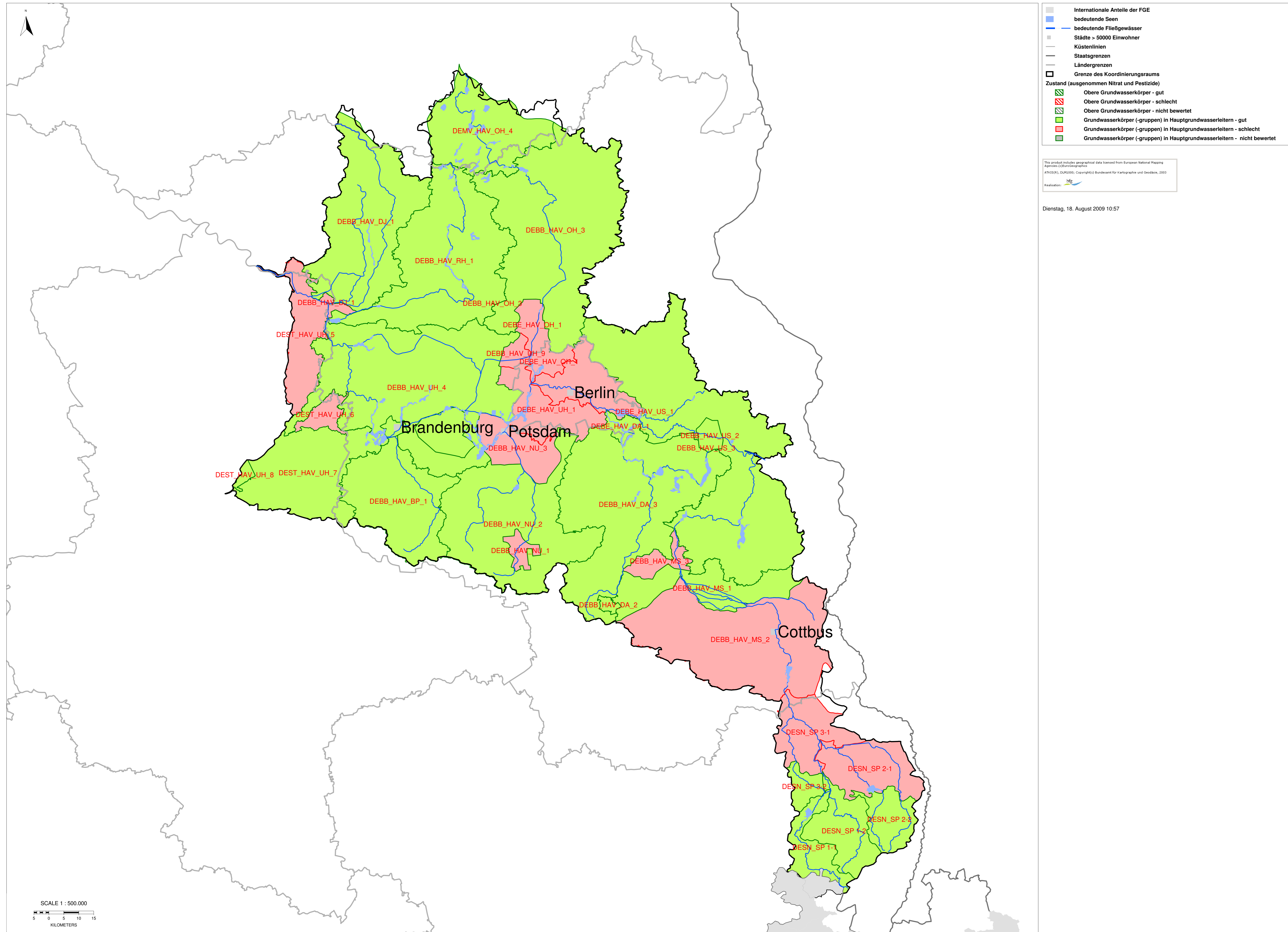
Koordinierungsraum Havel, Karte 4.6.3: Chemischer Zustand der Grundwasserkörper hinsichtlich der Schadstoffe nach Anhang II der Tochterrichtlinie Grundwasser und anderer Schadstoffe
